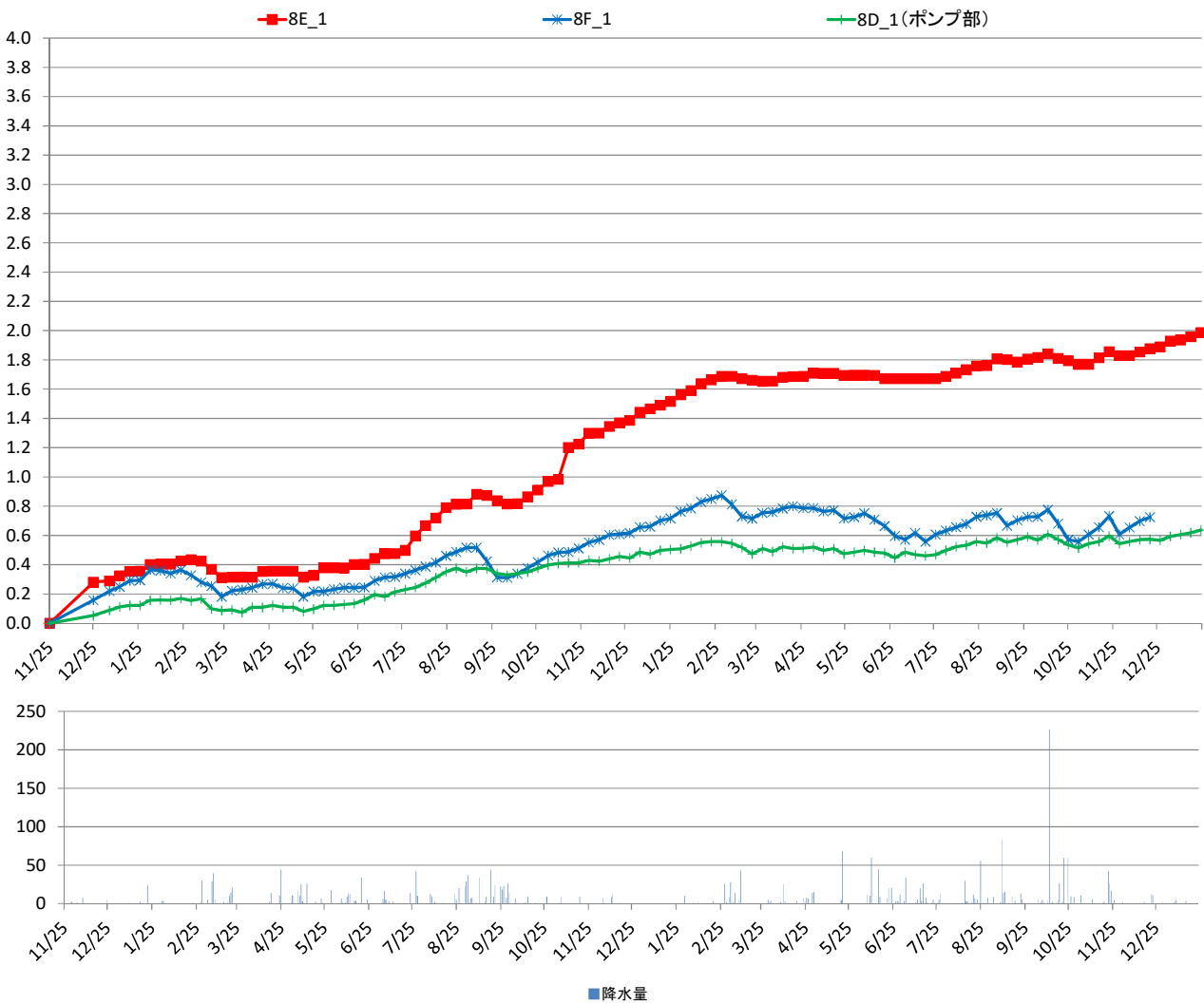
8丁目沈下 (G.L-cm)
