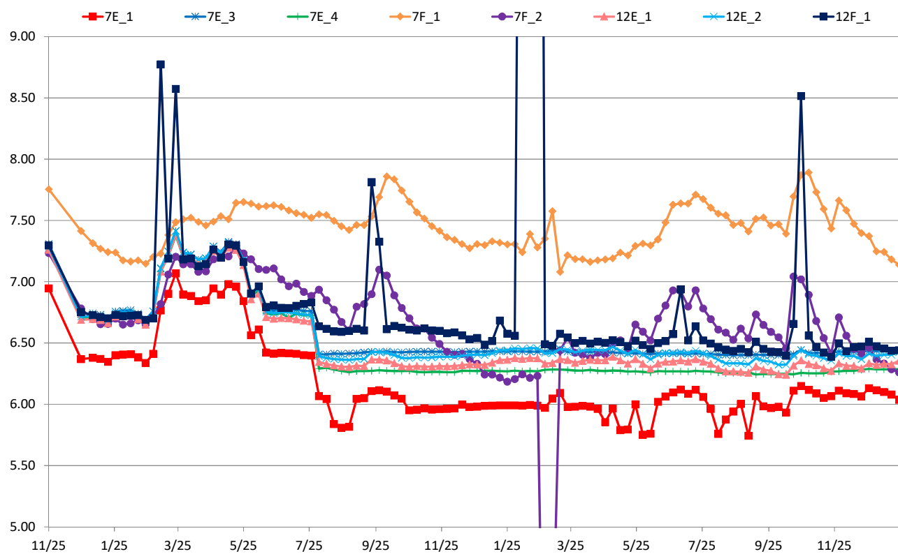
7・12丁目沈下 (G.L-cm)
