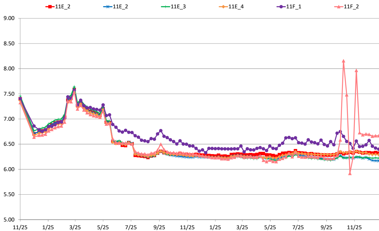
1 1丁目沈下 (G.L-cm)
