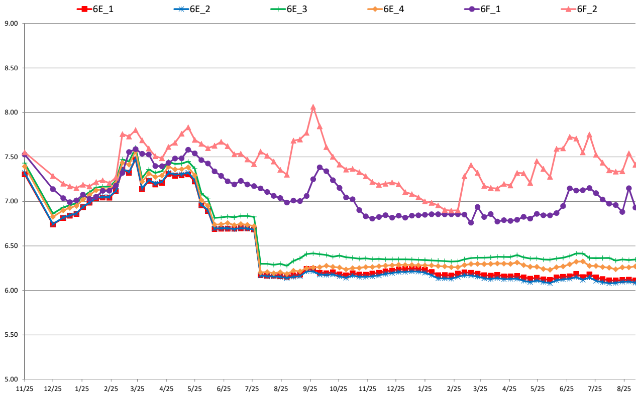
6丁目沈下 (G.L-cm)
