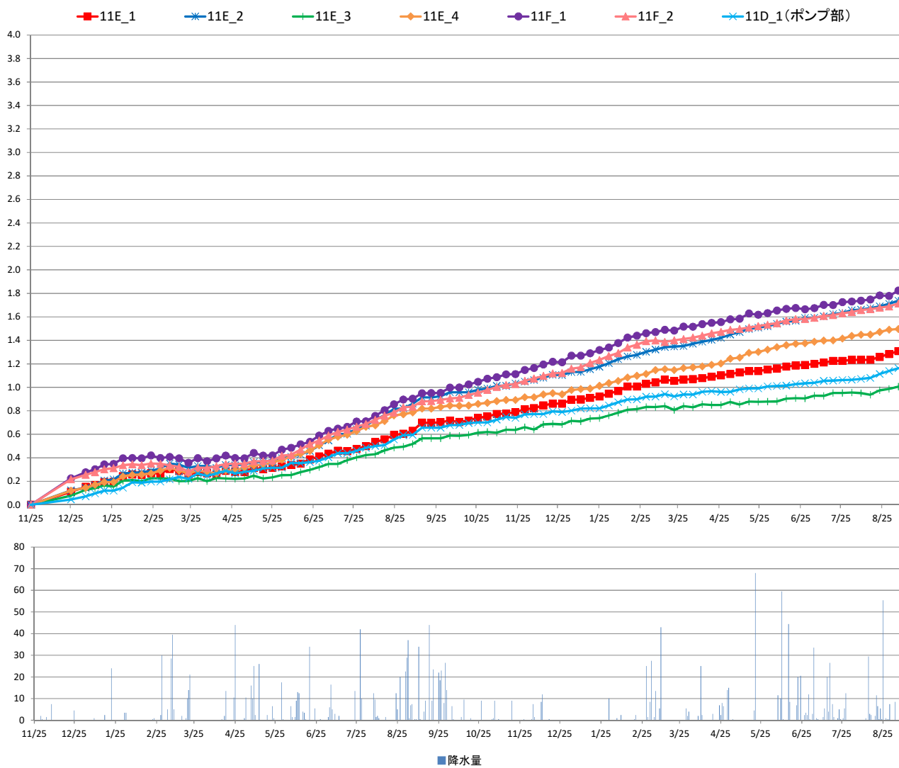
1 1 丁目沈下 (G.L-cm)
