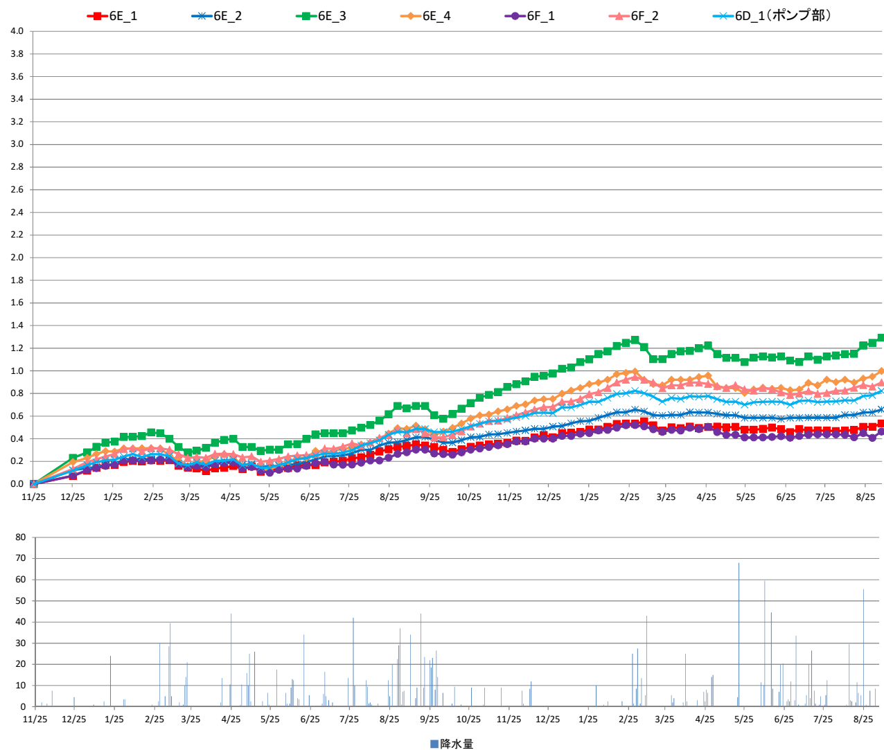
6丁目沈下 (G.L-cm)
