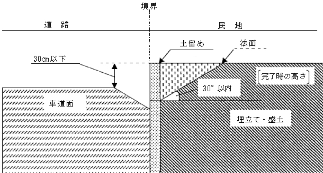
②用排水施設のない道路(例示 2)
