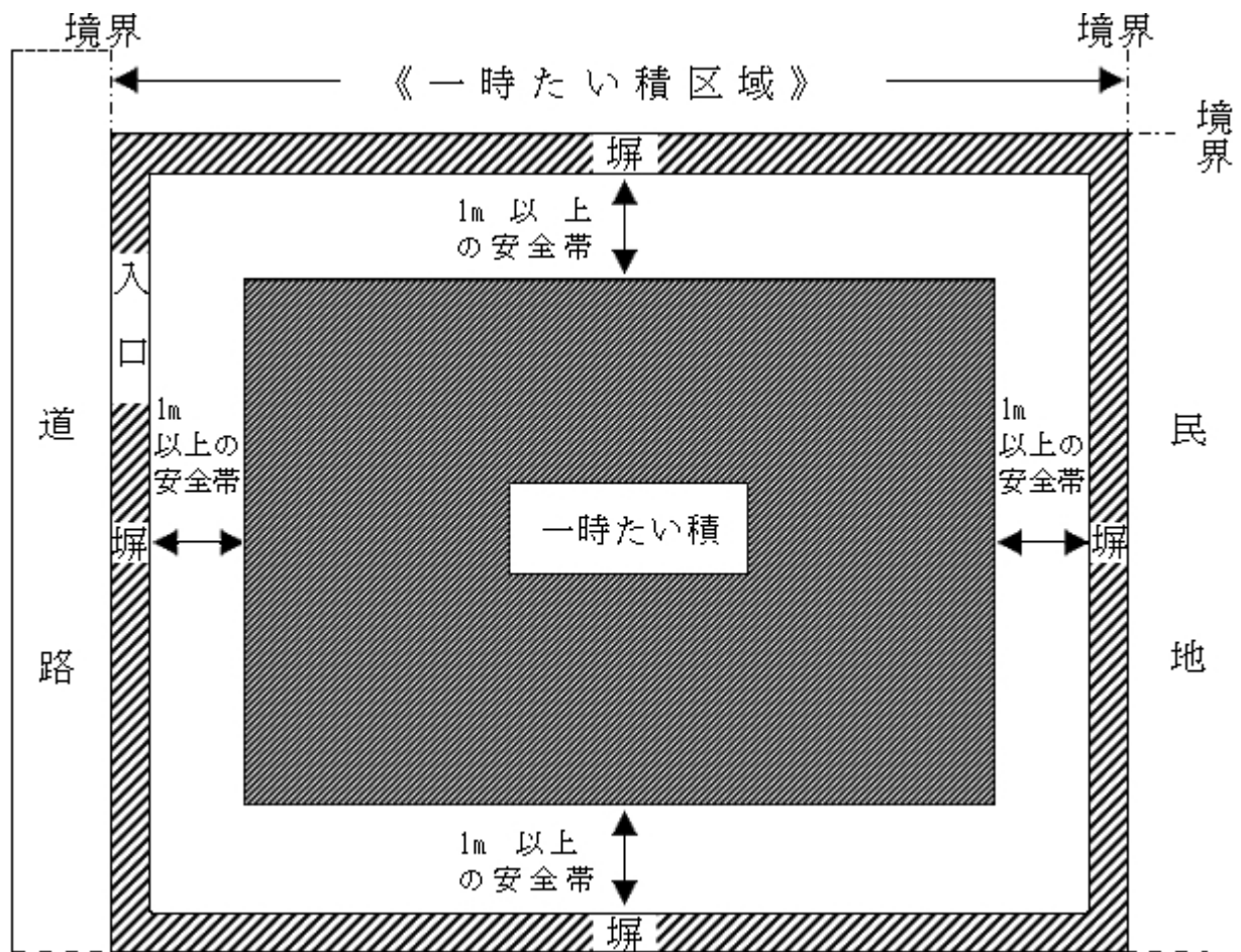
②平面図(例示 4)
