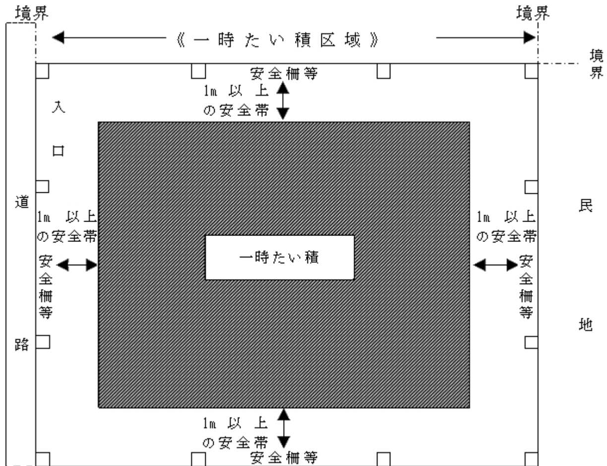
②平面図(例示 6)
